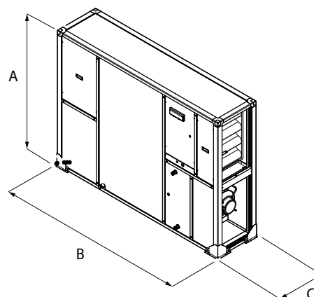
Installazione Verticale
