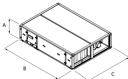
Installazione Orizzontale
